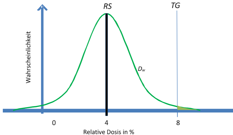
Abb. 4: Beispiel für die Bestimmung der Reaktionsschwelle RS mit TG = 8\% und s = 2\% mit einem Konfidenzintervall \alpha von 1,96 s. Die Kurve zeigt die angenommene Wahrscheinlichkeitsverteilung der wahren Dosis. Es ergibt sich eine Reaktionsschwelle von 4%.
