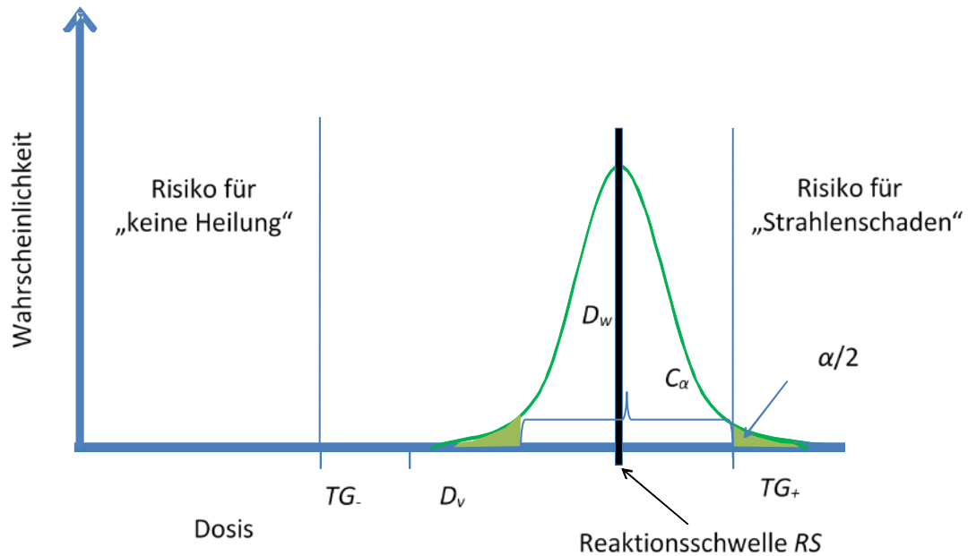
Abb. 3: Bestimmung der Reaktionsschwelle RS aus der oberen Toleranzgrenze TG_+ unter Berücksichtigung der Unsicherheit der gemessenen „wahren“ Dosis D_w . Innerhalb des Konfidenzintervalls liegen (1-\alpha)\% der Werte von D_w , außerhalb liegen \alpha\% der Werte. In dieser Grafik weicht die wahre Dosis von der verordneten Dosis D_v nach oben ab. Damit liegen im dargestellten Fall \alpha/2 der gemessenen Werte oberhalb der Toleranzgrenze und die Reaktionsschwelle ist erreicht.
