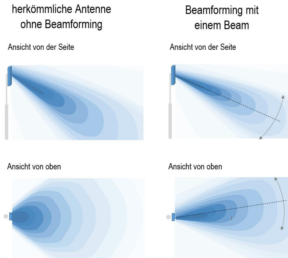
Abb. 1-2: Schematische Darstellung des Beamformings anhand eines Vergleichs der (statischen) Abstrahlcharakteristik einer herkömmlichen Antenne (links) und einer MIMO-Antenne bei Aussendung eines Beams (rechts). Dunkle Bereiche kennzeichnen höhere Feldstärken, helle Bereiche kennzeichnen geringere Feldstärken. Die Hauptsenderichtung und die Form der Beams ist bei MIMO-Antennen dynamisch (softwaregesteuert) veränderlich (in der Abbildung angedeutet durch Pfeile).
